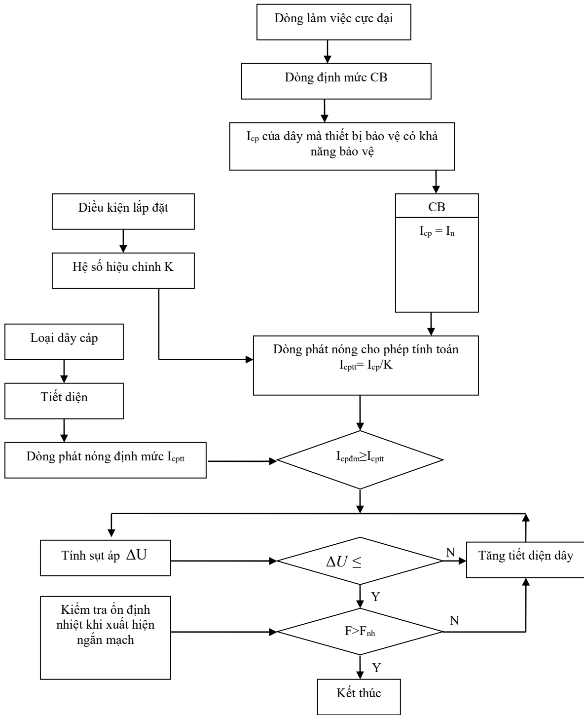
Thủ tục đầy đủ lựa chọn dây/cáp mạng hạ áp
