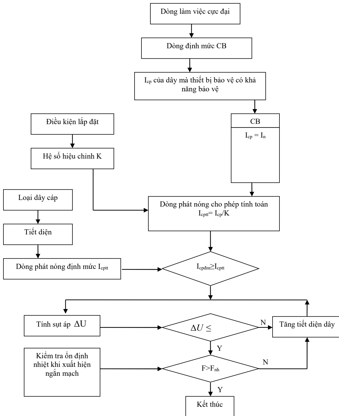
Thủ tục dây đủ lựa chọn dây/cáp mạng hạ áp
